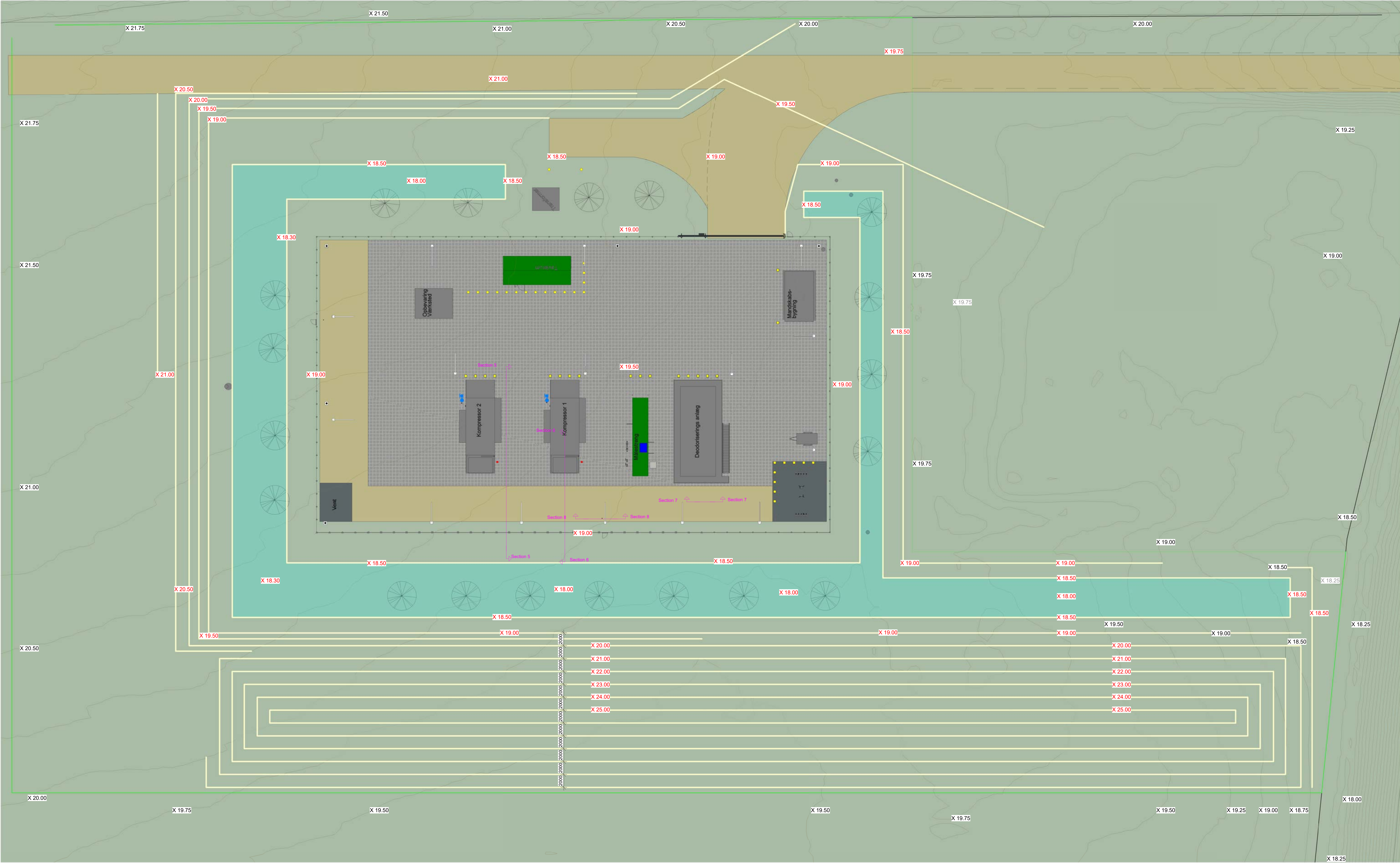
Belægningsplan Mål 1 : 200
